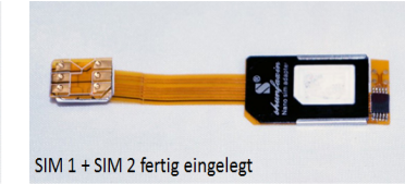
Dual SIM Adapter wie abgebildet in den mod. SIM Tray einsetzen
